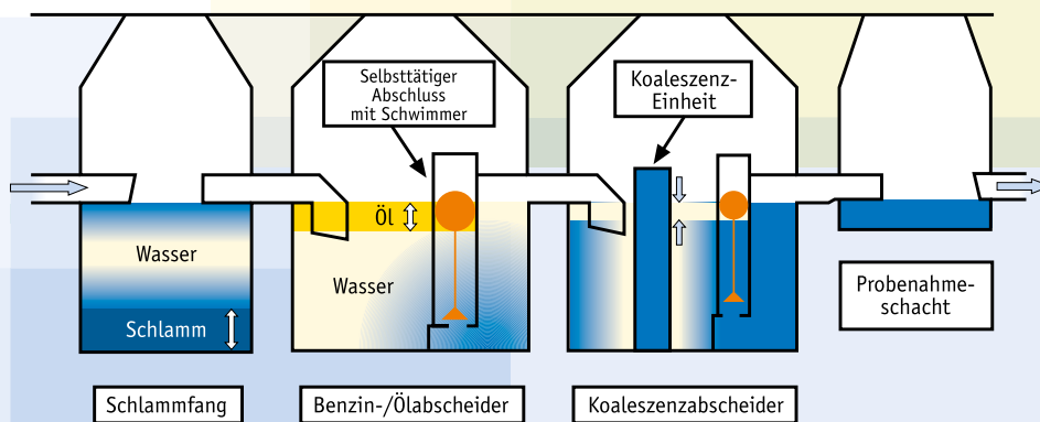
Komponenten einer großen Leichtflüssigkeitsabscheideranlage nach DIN 1999
